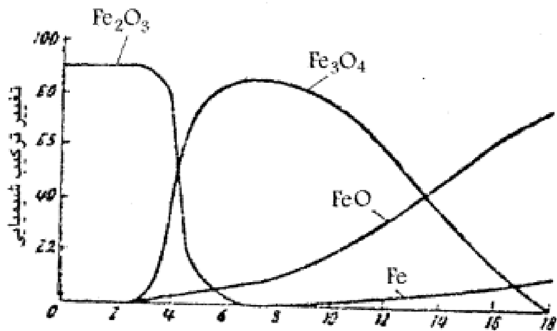
شکل ۳-۴: تغییرات ترکیب شیمیایی بر حسب درصد مصرف کربن در پخت کلوخه [۲۴]
