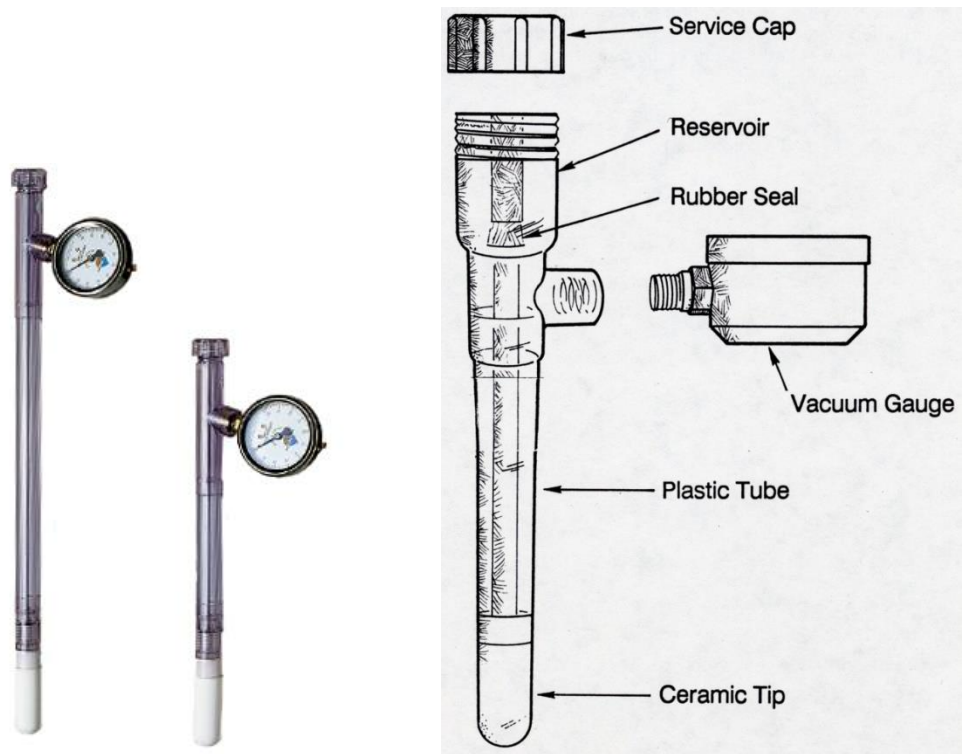
تانسیومتر فلزی
