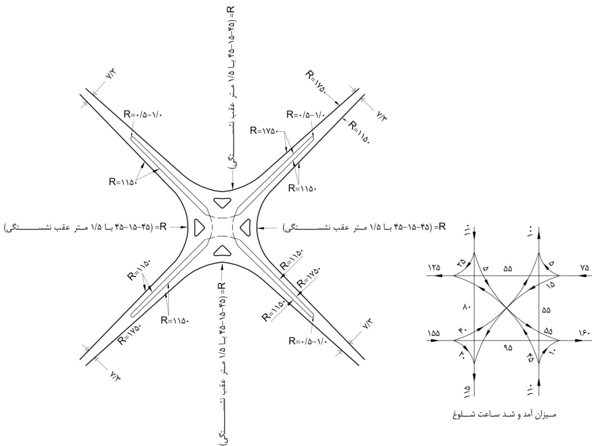
ت - چهارراه با جزیره‌های ترافیکی بدون خط کمکی (تعمیر شده)
