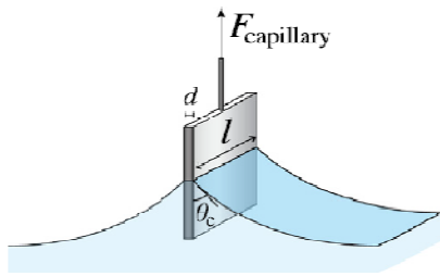
Wilhelmy plate
