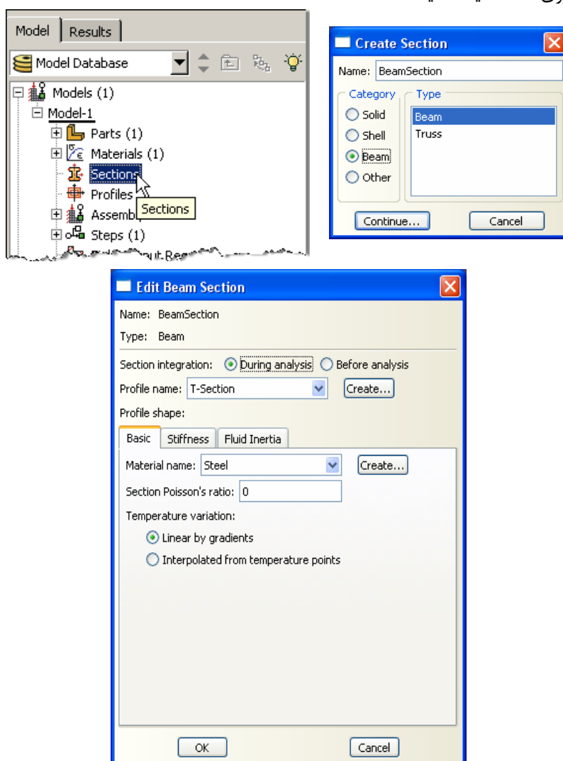
شکل ۱۰-۹- مراحل تعریف سطح مقطع اعضای پل
