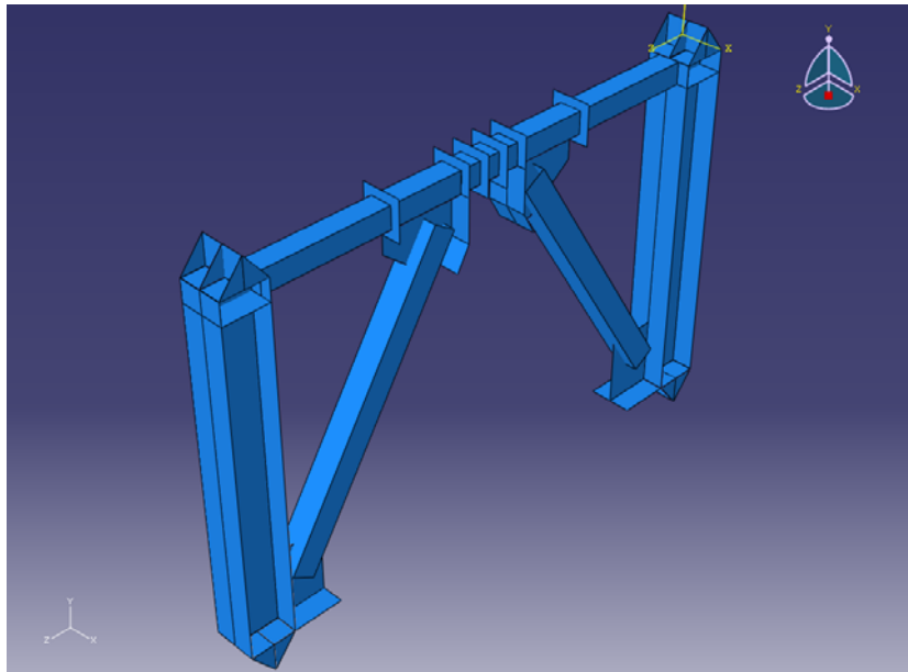
شکل ۸-۹۶- قاب واگرای ساخته شده در ماژول Assembly
