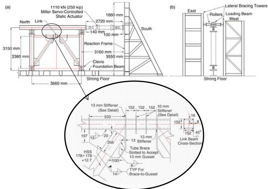
شکل ۸-۱- هنده و موقعیت قاب واگرای مورد نظر
