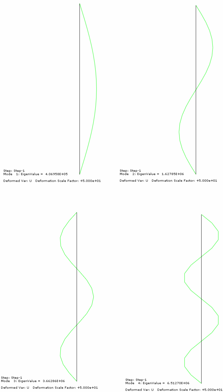
شکل ۵-۲۸- شکل مودهای اول تا چهارم ستون
