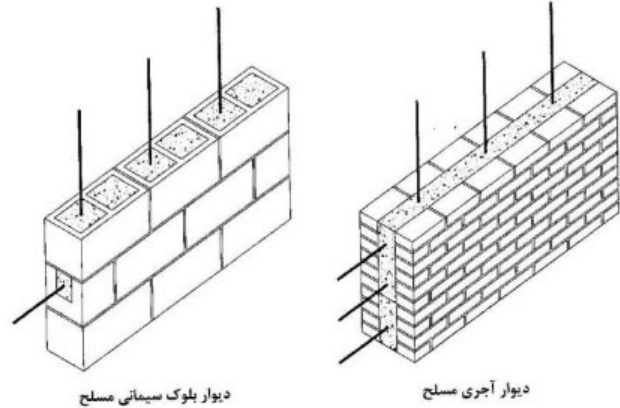
شکل ۸-۴-۱ نمونه‌هایی از دیوارهای بنایی مسلح
