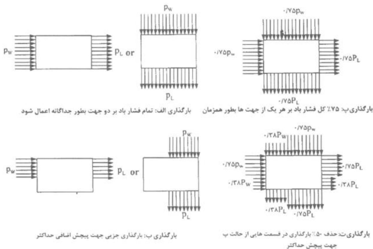
شکل ۶-۱۰-۸ بارگذاری باد کامل و جزئی
